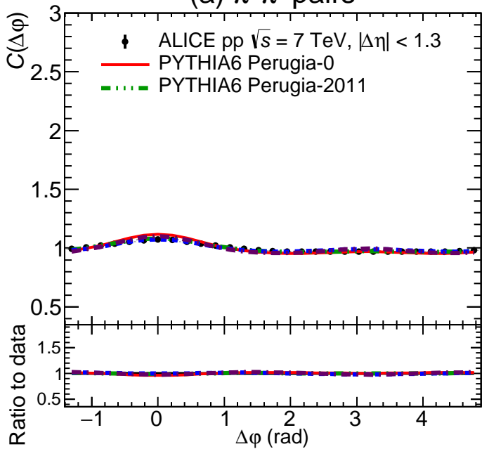
(a) \pi^+\pi^- pairs
