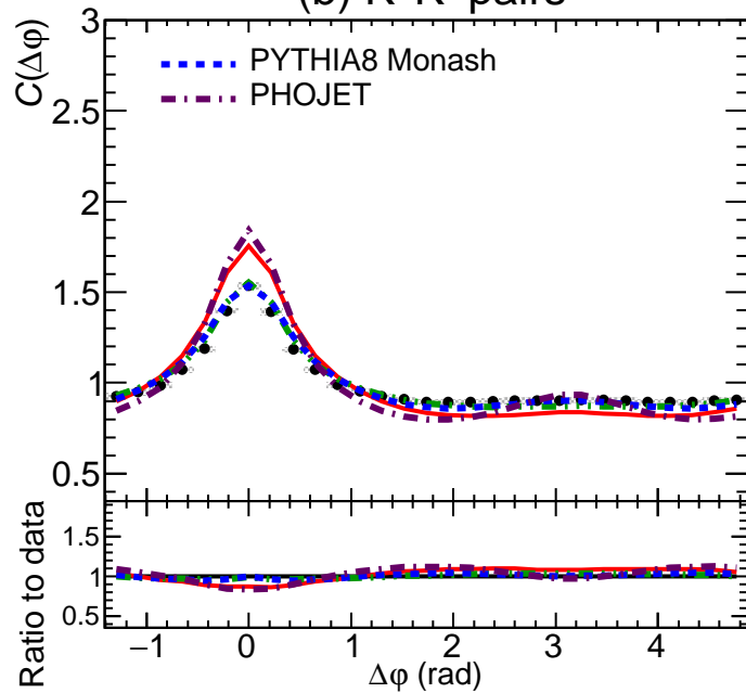
(b) K^+K^- pairs
