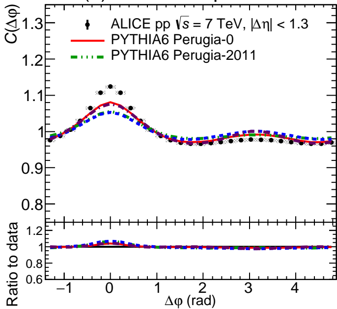
(a) \pi^+\pi^+ + \pi^-\pi^- pairs
