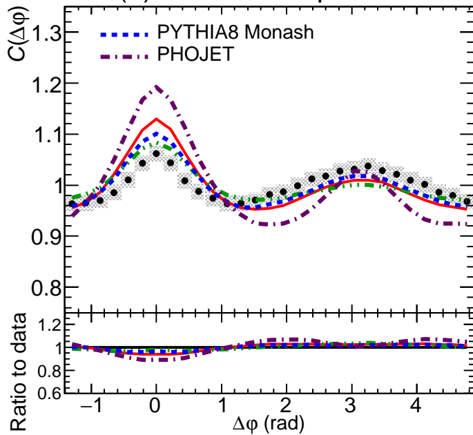
(b) K^+K^+ + K^-K^- pairs
